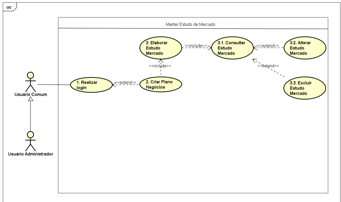
Figura 8. Diagrama do caso de uso Manter Estudo de Mercado
