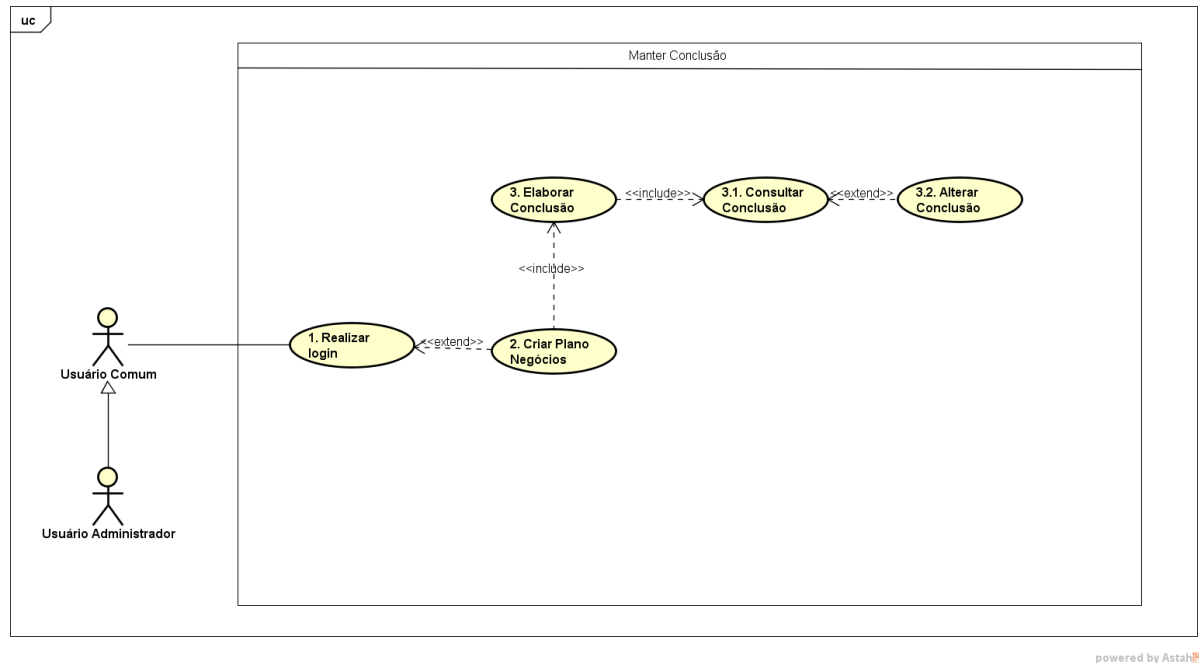
Figura 12. Diagrama do caso de uso Manter Conclusão
